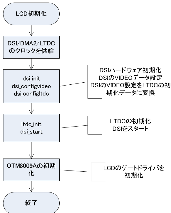
図 4.3.6.3.1 LCD 初期化
