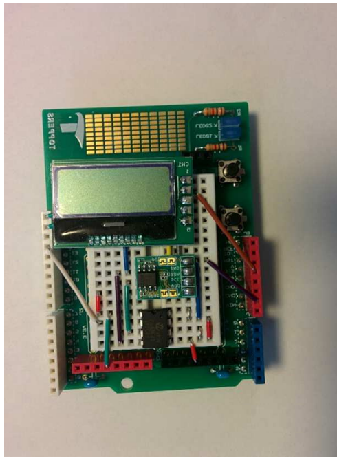
I2C プロトタイプシールド
