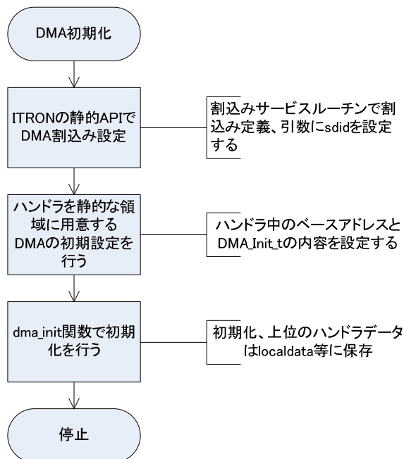
図 4.1.4.3.1 DMA 初期化
