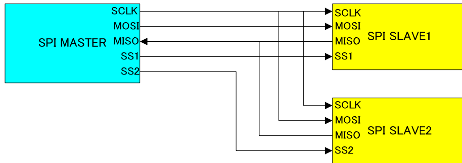
図 4.2.3.1 SPI 接続図
